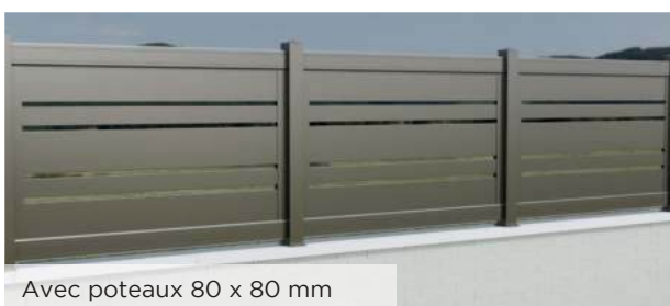
Coloris RAL 7006 FT - avec poteau 80 x 80 mm Dimensions maxi. entre poteaux : 2000 mm pour poteaux de 80 x 80 mm, 1500 mm pour poteaux de 70 x 70 mm
