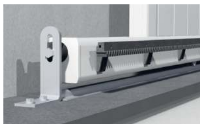
Rail inox + Butée + Roulette pour portail coulissant composée de : • chape alu (couleur portail) • galet inox + Crémaillère en nylon armé pour motorisation
