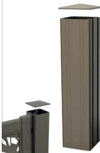
SCELLEMENT 400 MM 188 x 188 mm Rainuré . Alu à sceller
